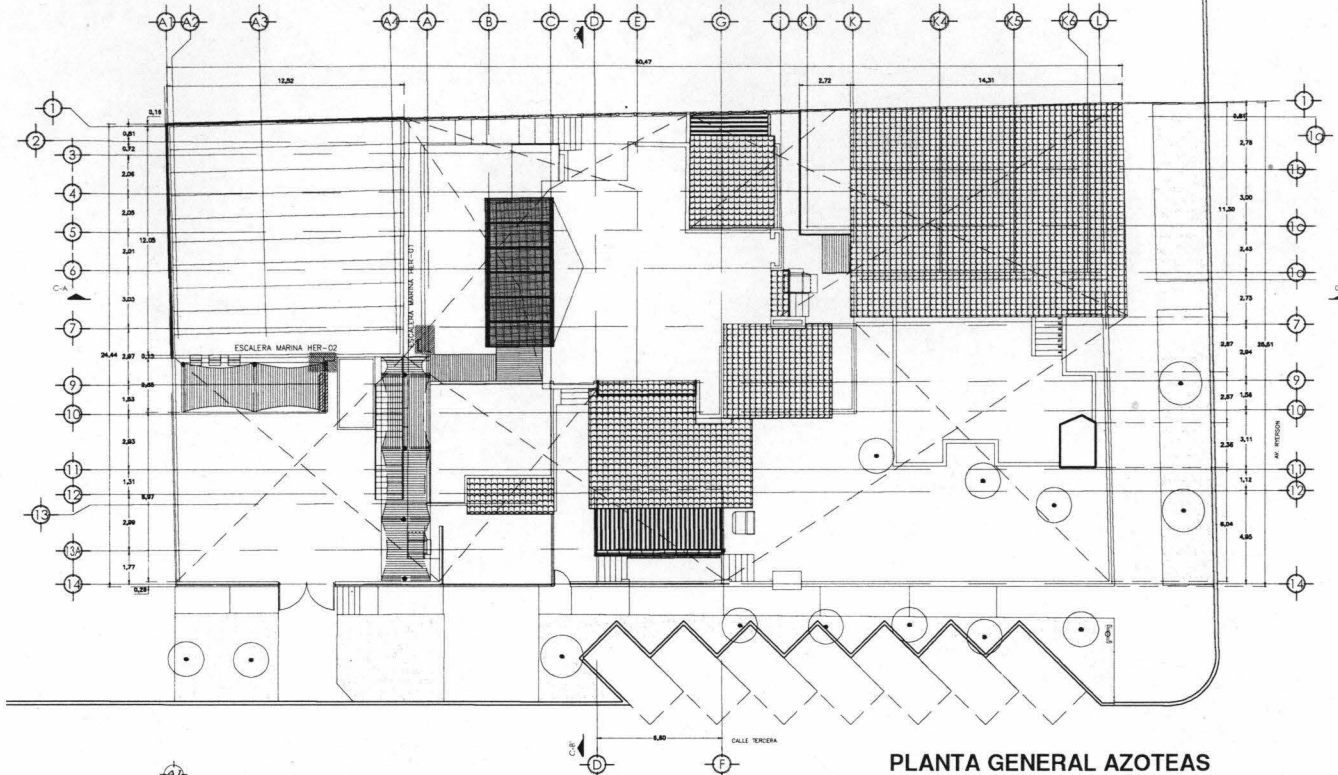
PLANTA GENERAL AZOTEAS
