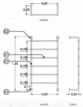
ESCALERA MARINA HER-01
