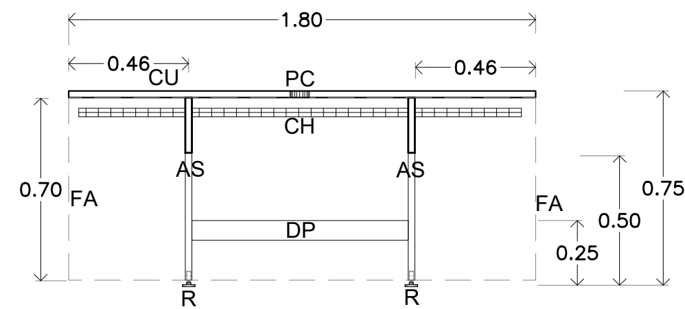
ALZADO FRONTAL ESCALA 1:30 PZAS. 4
