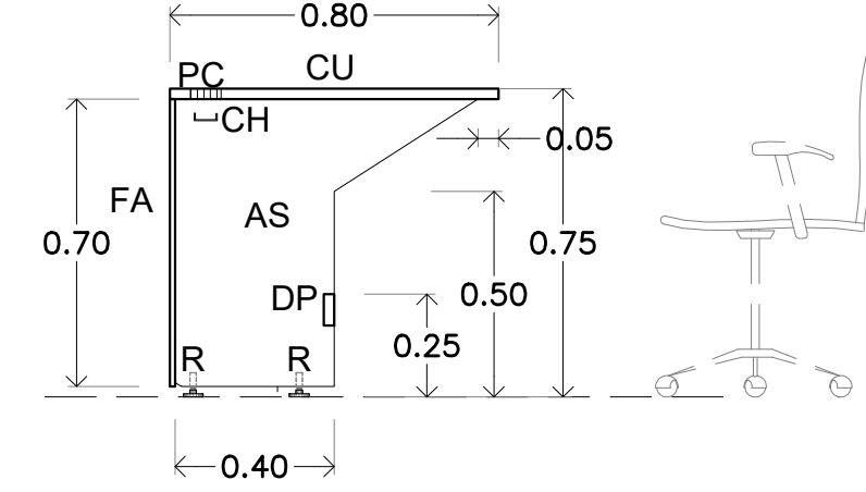
CORTE TRANSVERSAL ESCALA 1:30 PZA. 1
