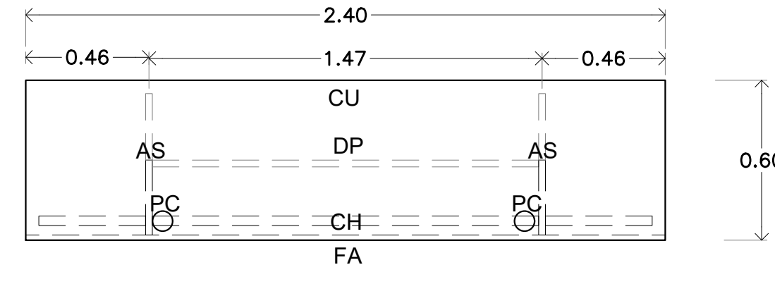
PLANTA ESCALA 1:30 PZA. 1
