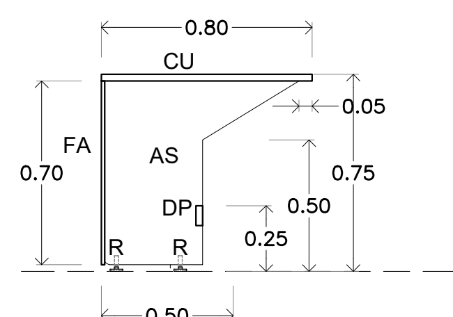
ALZADO LATERAL ESCALA 1:30 PZA. 2
