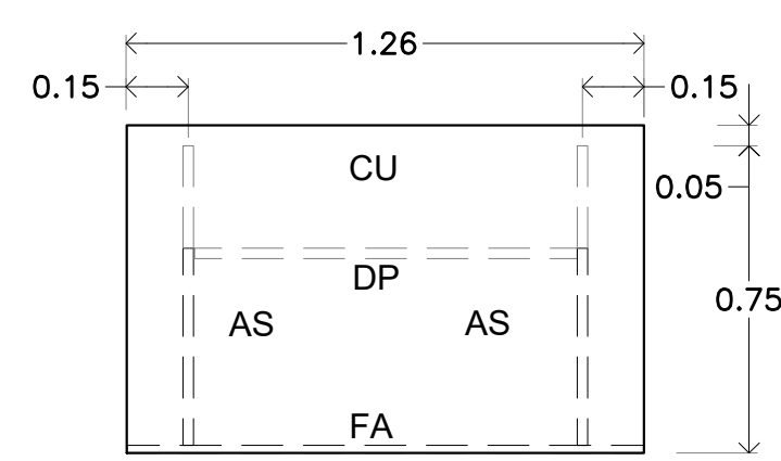
PLANTA ESCALA 1:30 PZA. 2
