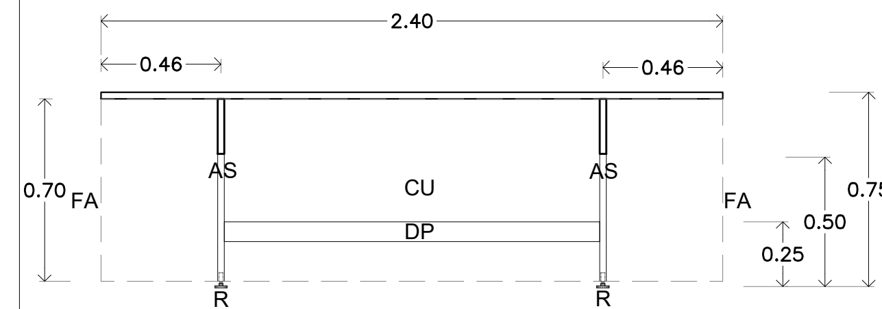
ALZADO FRONTAL ESCALA 1:30 PZAS. 8
