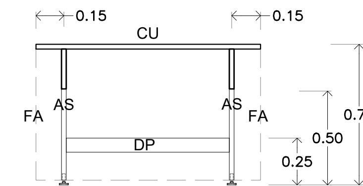
ALZADO FRONTAL ESCALA 1:30 PZA. 2
