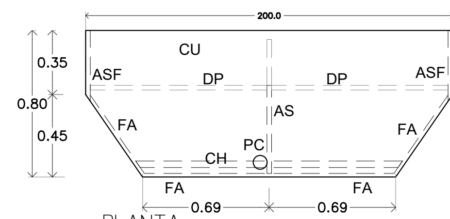
PLANTA ESCALA 1:30 PZA. 1
