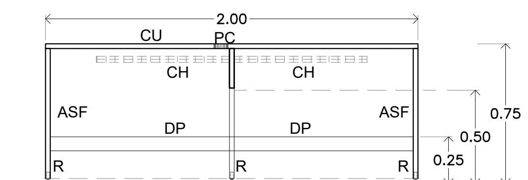
CORTE LONGITUDINAL ESCALA 1:30 PZA. 1
