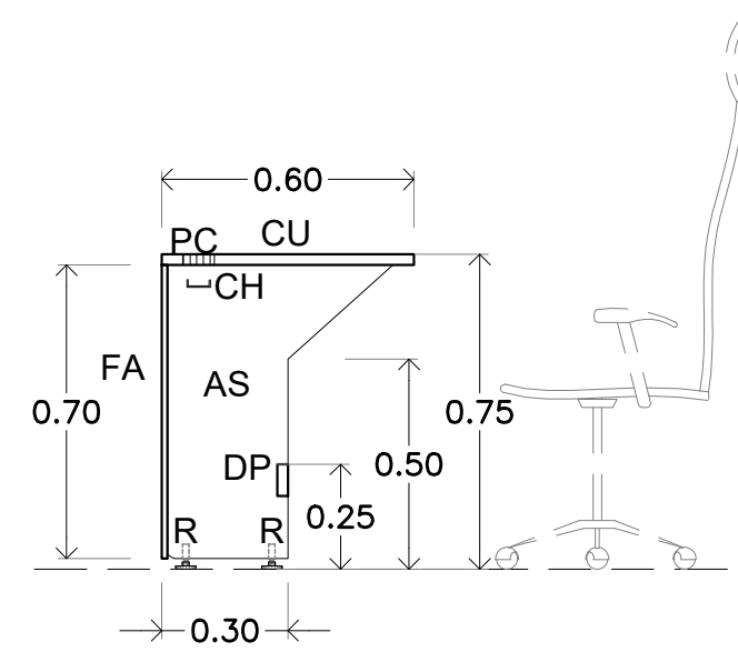
ALZADO LATERAL ESCALA 1:30 PZAS. 4
