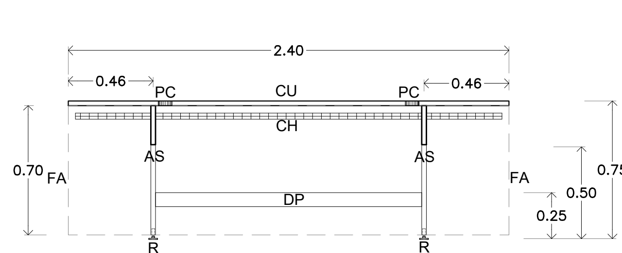
ALZADO FRONTAL ESCALA 1:30 PZA. 1
