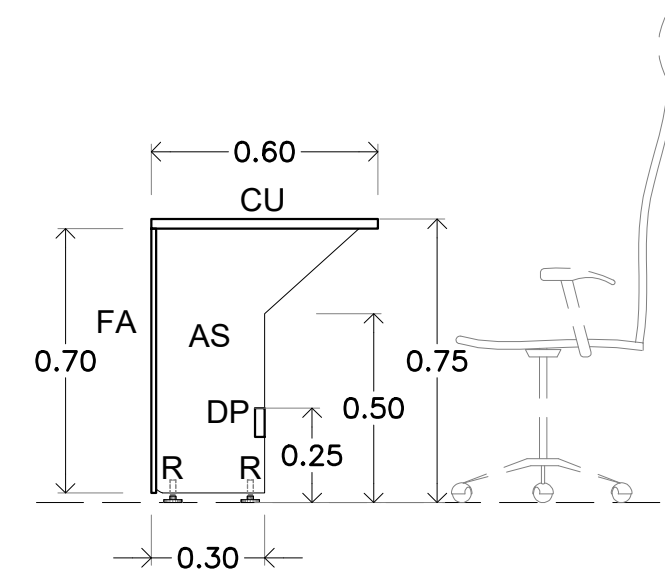
ALZADO LATERAL ESCALA 1:30 PZAS. 8
