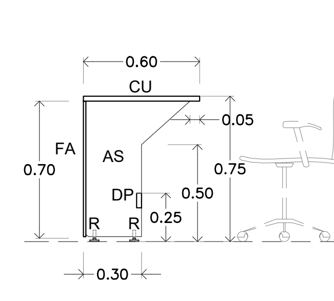
ALZADO LATERAL ESCALA 1:30 PZA. 2
