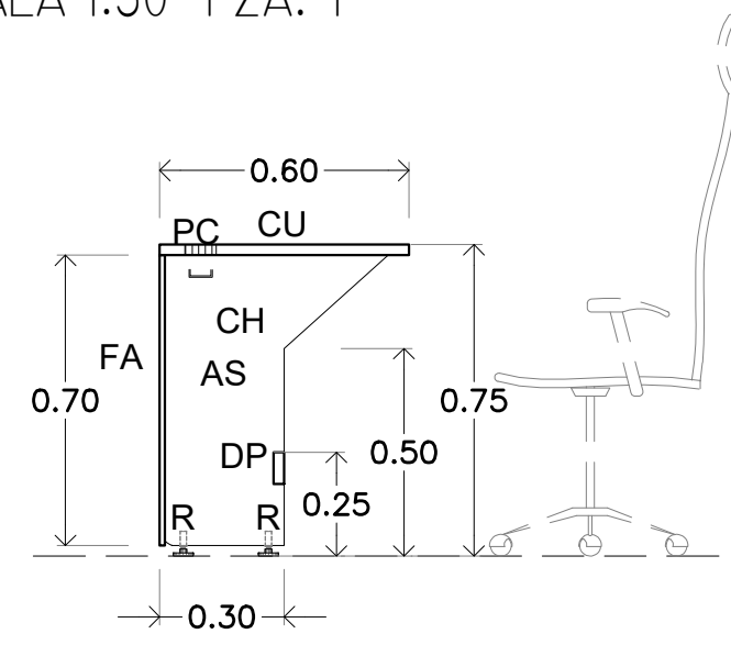
ALZADO LATERAL ESCALA 1:30 PZA. 1
