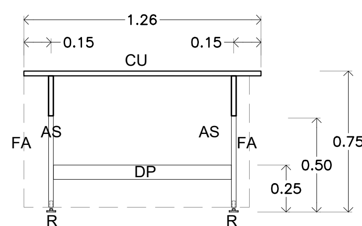
ALZADO FRONTAL ESCALA 1:30 PZA. 2
