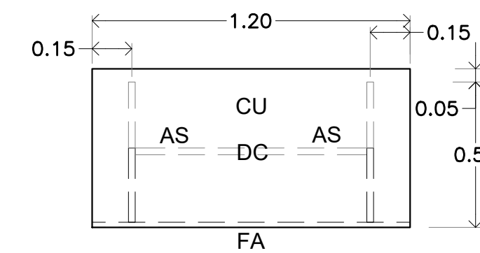
PLANTA ESCALA 1:30 PZA. 2
