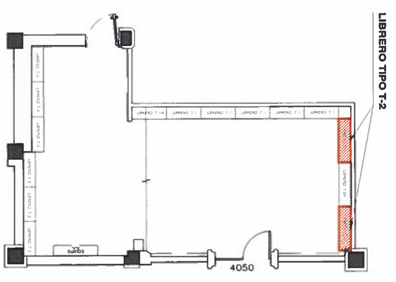
PLANTA DE UBICACIÓN LIBRERO TIPO T-2
