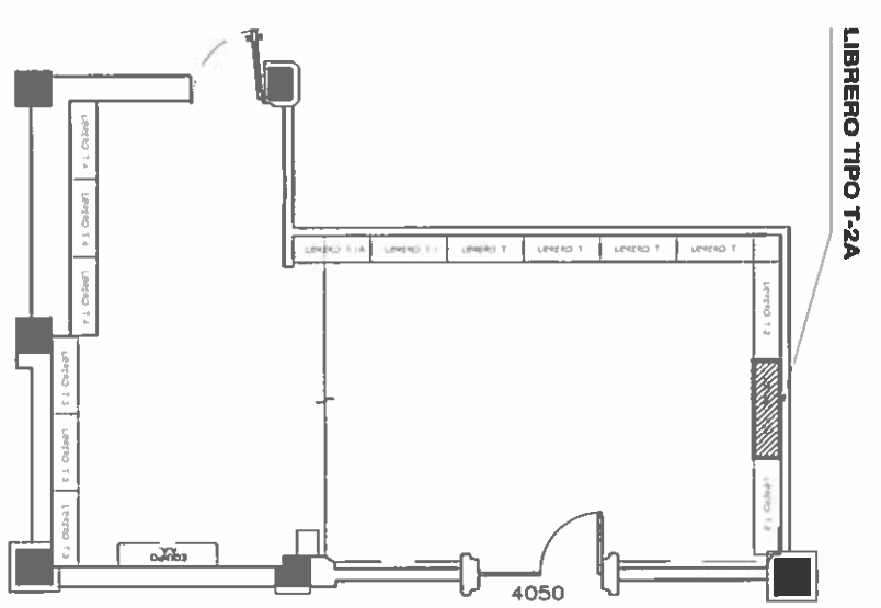
PLANTA DE UBICACIÓN LIBRERO TIPO T-2A
